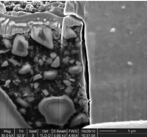
FIGURA 3. Sin ningún pretratamiento de la superficie, la interfaz de unión entre la resina y el óxido de circonio revela espacios muy abiertos y una adhesión limitada.
